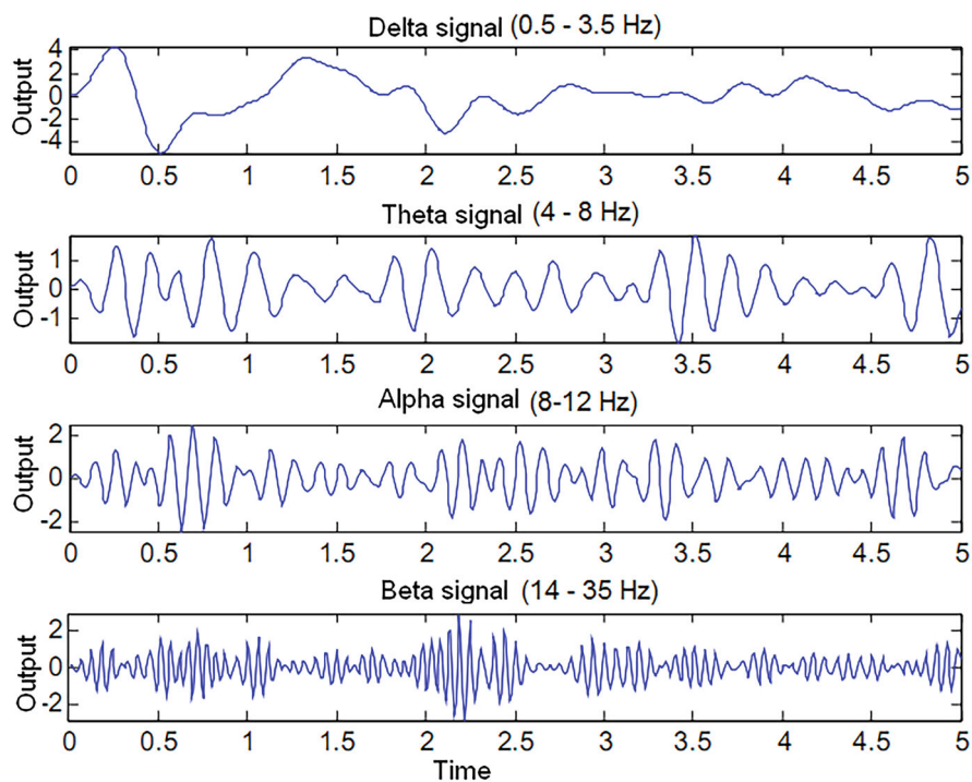
Fig. 9.2 EEG signals
